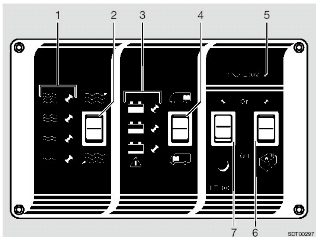
Fig. 1 Panneau de contrôle et de commande LT 300
